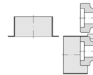
Kastensickenwalzen SK
